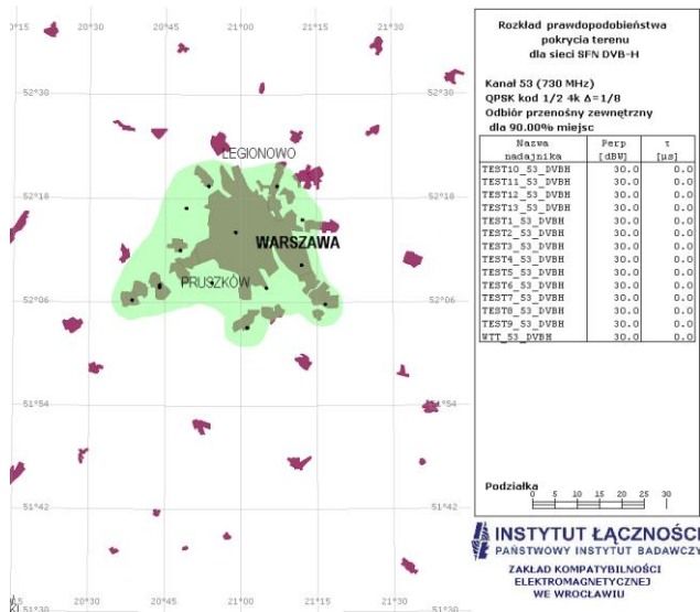
Rys. 2. Zasięg sieci SFN DVB-H 1kW
