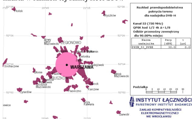
Rys. 1. Zasięg stacji DVB-H ERP=1kW, PKiN
